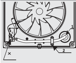
Рис. 3 AEON / SLIM
