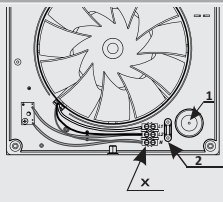
Рис. 2 AURA 6 / SILENT 6
